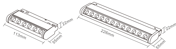
磁吸旋转格栅灯系列 48V Magnetic Adjustable Grille Light Series
