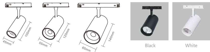
磁吸轨道灯系列 48V Magnetic Track Light Series
