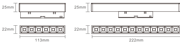
磁吸格栅灯系列 48V Magnetic Grille Light Series
