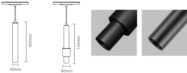
磁吸吊线灯系列 48V Magnetic Pendant Light Series
