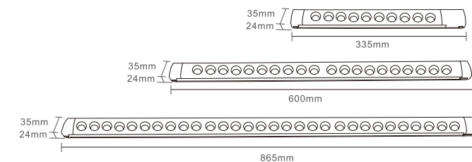
35磁吸格栅灯系列 48V Magnetic Grille Light Series
